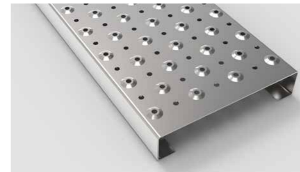
Type AP 2 - 50 avec drainage (MAA) Type AP 3 - 50 avec drainage (MAA) Dôme gaufré avec perforation Ø 8 mm sur 3 mm de hauteur. Perforation de drainage plate de Ø 8 mm, toutes deux en quinconce de 50 mm c.t.c.
